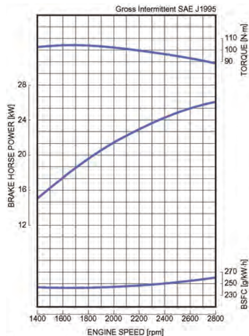
D1703 Performance Curves
